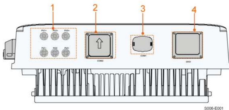
Figura 5-1 Terminais
